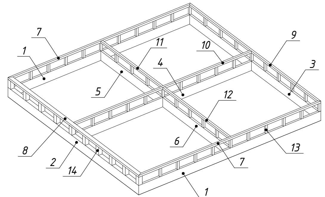
Изометрия представлена с тыльной стороны.
